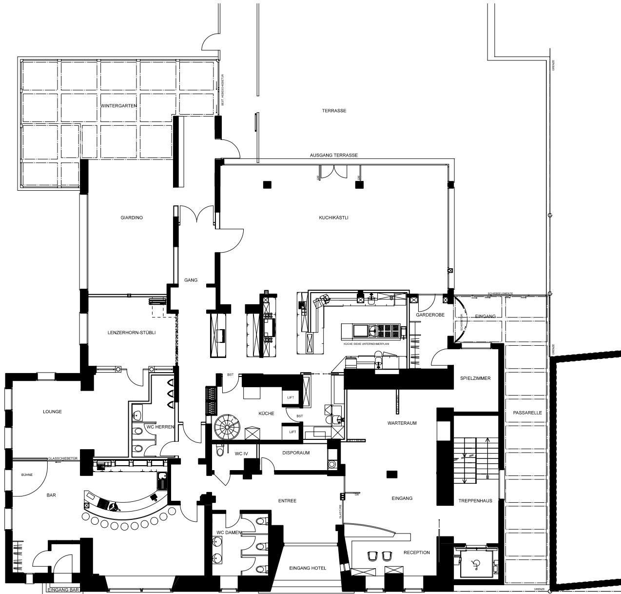
HOTEL LENZERHORN GRUNDRISS EG BEST. LENZERHORN (LEER) DATUM: 21.03.06 GEZ. sj
